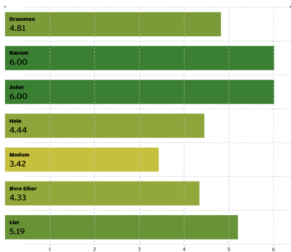
KLNO3 Endring i klimagassutslipp (tonn CO2 ekvivalenter) fra veitrafikk i kommunen siste fire år
