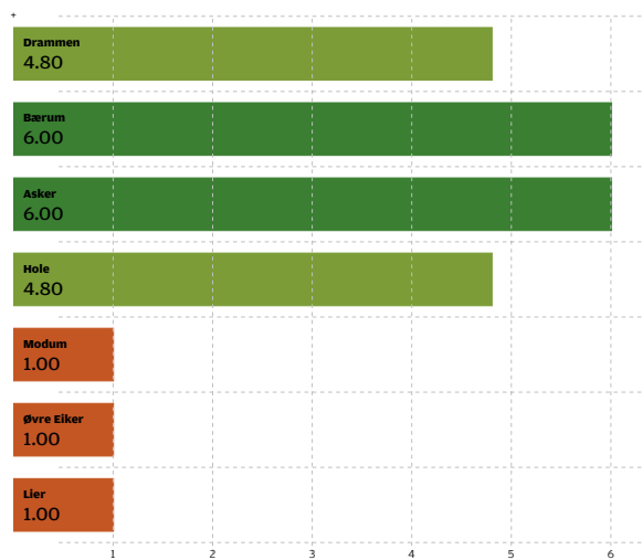
KLNO4 Hvor mange av de siste fire årene kommunen har søkt om midler fra Klimasats
