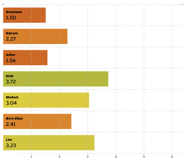
KLNO5 Antall offentlige ladepunkt for elbiler per 1000 innb.
