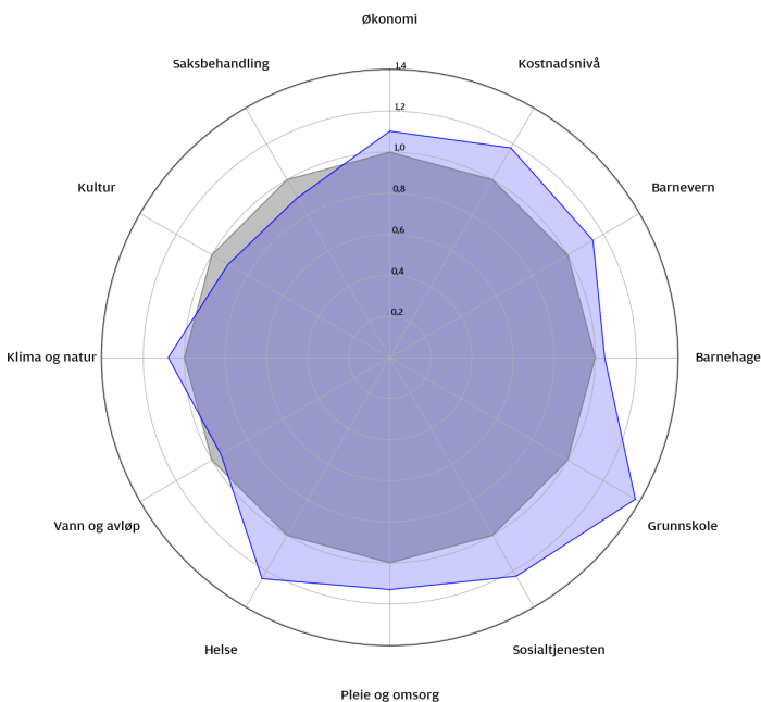
FIGUR 1: Radardiagrammet viser hvordan Lier skårer i forhold til landsgjennomsnittet innenfor hver sektor. Grått område definerer gjennomsnittskommunen (0% for alle sektorer).
